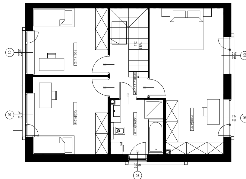
RZUT PIĘTRA LOKAL A4
