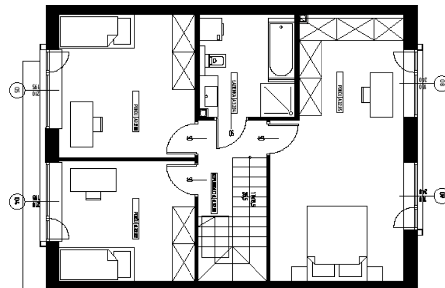
RZUT PIĘTRA LOKAL A3
