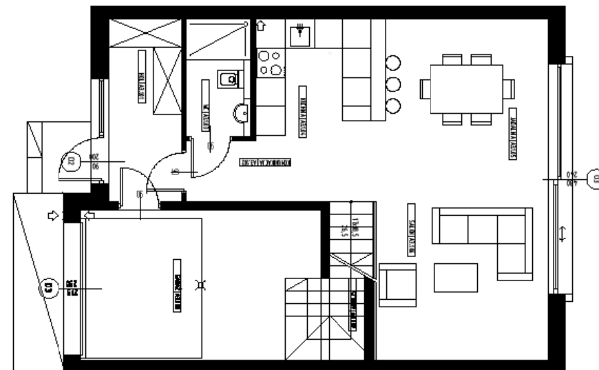
RZUT PARTERU LOKAL A3
